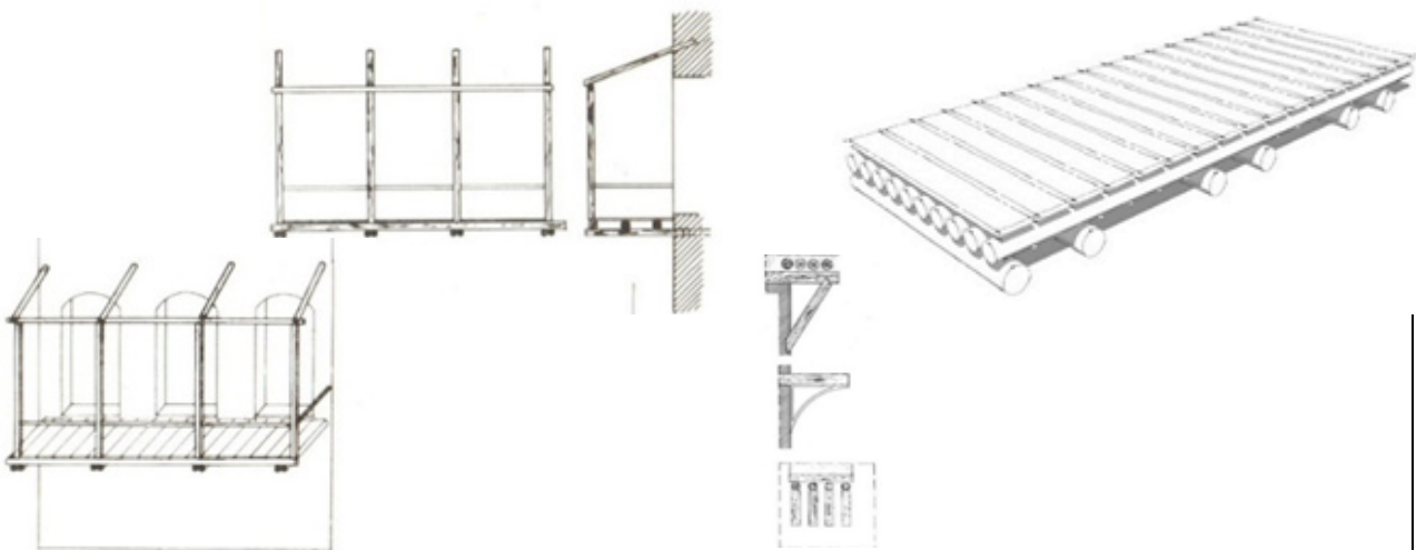
شکل ۳ تا ۶. ساختار و اسکلت کلی شناسیرها در بندر بوشهر (مخلصیان، ۱۳۹۰، ۸۴) Figure 3 to 6. The General Structure and Body of Shanshirah in Bushehr Port
