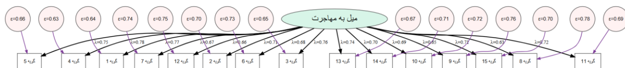
شکل ۲. نمودار تحلیل عاملی تأییدی پرسش نامه میل به مهاجرت
