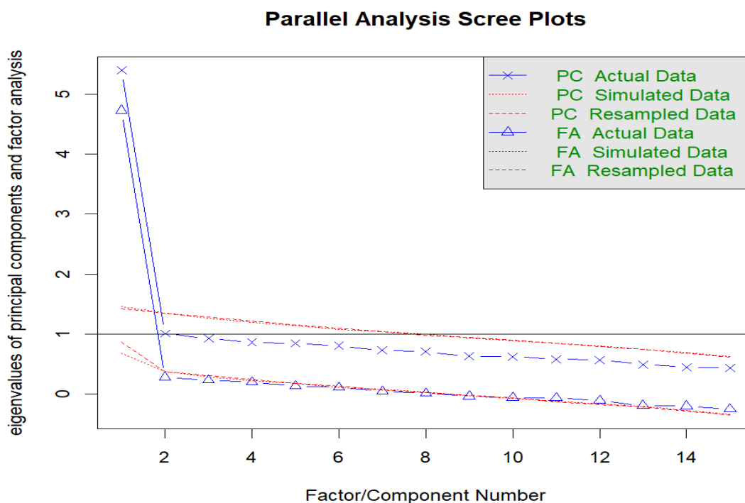
شکل ۱. نتایج آزمون اسکری تحلیل موازی
