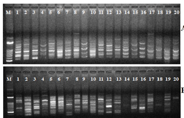
شکل ۱: الکتروفورز محصول PCR نشانگر REP-PCR (A) و نشانگر BOX-PCR (B) DNA باکتری‌های مورد مطالعه (حرف M و اعداد ۱ الی ۲۰ به ترتیب بیانگر نشانگر ۱۰۰bp و شماره باکتری‌های مورد مطالعه می‌باشد).
