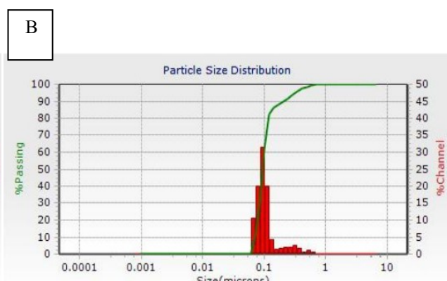
شکل ۲: تست DLS اندازه نانوذرات اکسید روی (A) و نانوذرات اکسید گرافن (B).
