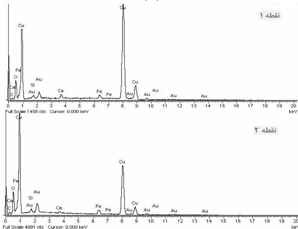
شکل 1- (الف) تصویر میکروسکوپی الکترونی روبشی از نمونه بتنی پوشش داده شده با جریان مستقیم و محلول الکترولیت بدون ملاس؛ (ب) آنالیز EDS در دو نقطه شماره گذاری شده.
