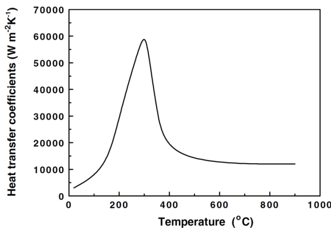
شکل (۲) - تغییرات ضریب همرفتی فواره آب مورد استفاده در آزمون استاندارد سختی پذیری با دما [۱۳]
