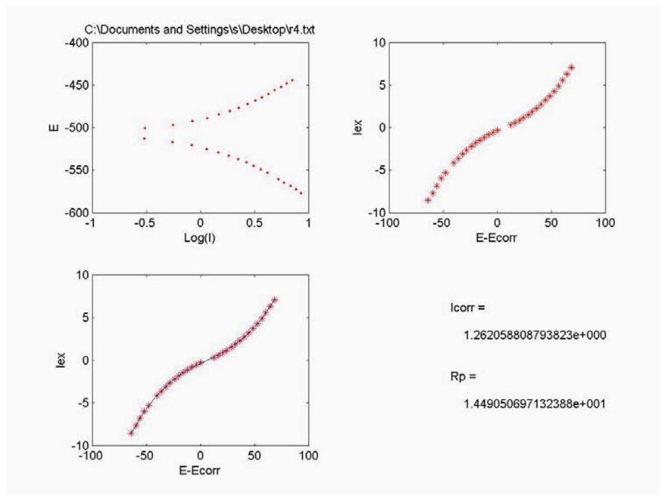
شکل ۷- شمای خروجی نرم‌افزار EKMS
