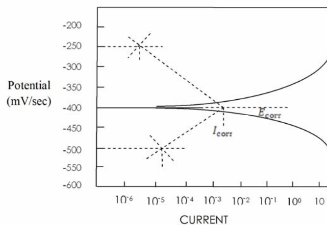
شکل ۸- شماتیک منحنی کلی پلاریزاسیون که در رسم آن از فرض‌های ساده شونده استفاده شده است. [۱۶]
