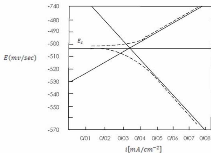
شکل ۴- منحنی پلاریزاسیون آهن آرمکو در اسید سولفوریک ۱ نرمال، در دمای ۲۵ [۱۳]
