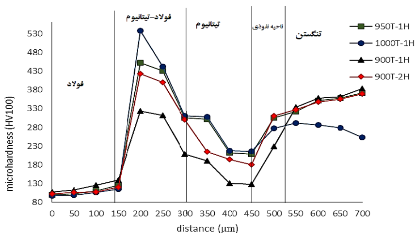
شکل ۸- پروفیل میکروسختی نمونه‌های اتصال یافته در دماها و زمان‌های مختلف
