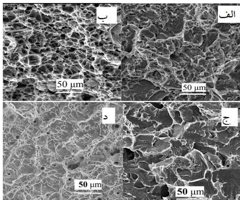
شکل ۹- تصاویر SEM سطح شکست اتصال در نمونه اتصال داده شده در: الف) دمای °C ۹۰۰ به مدت ۱ ساعت (900T1H)، ب) دمای °C ۹۵۰ به مدت ۱ ساعت (950T1H)، ج) دمای °C ۱۰۰۰ به مدت ۱ ساعت (1000T1H) و د) دمای °C ۹۰۰ به مدت ۲ ساعت (900T2H)
