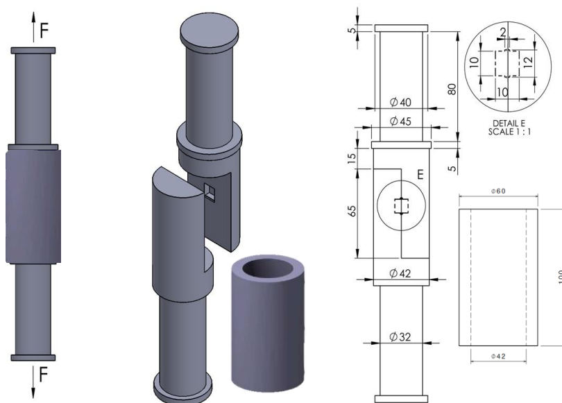
شکل ۲- طرحواره فیکسچر ارزیابی استحکام برشی اتصال
