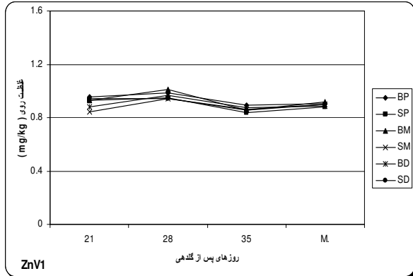
شکل ۲- منحنی روند تجمع عناصر ماکرو و میکرو مغذی در بخش‌های مختلف سنبله و سنبلیچه ارقام گندم در روزهای پس از گل‌دهی (V1 رقم مهدوی، V2 رقم فلات، BP و SP به ترتیب دانه‌های بزرگ و کوچک بخش پایینی سنبله، BM و SM به ترتیب دانه‌های بزرگ و کوچک بخش میانی سنبله، BD و SD به ترتیب دانه‌های بزرگ و کوچک بخش بالایی سنبله، Ca، K، Mn و Zn به ترتیب غلظت عناصر پتاسیم، کلسیم، منگنز و روی می‌باشند).
