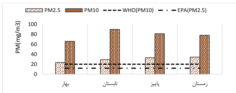
شکل ۴- تغییرات میانگین فصلی غلظت ذرات معلق (PM 2.5 و PM 10 ) در شهر تهران طی سال‌های ۹۹-۱۳۹۲
