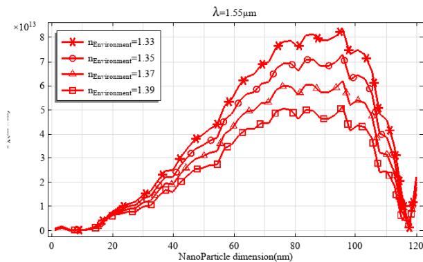
شکل (۹): تغییرات نیروهای تله‌انداز در محیط‌های با ضریب شکست ۱/۳۳ و ۱/۳۵ و ۱/۳۷ و ۱/۳۹ برحسب ابعاد ذرات پلی‌استایرن و در طول موج ۱/۵۵ میکرومتر در راستای x به ازای شعاع‌های مختلف ذرات پلی‌استایرن.
