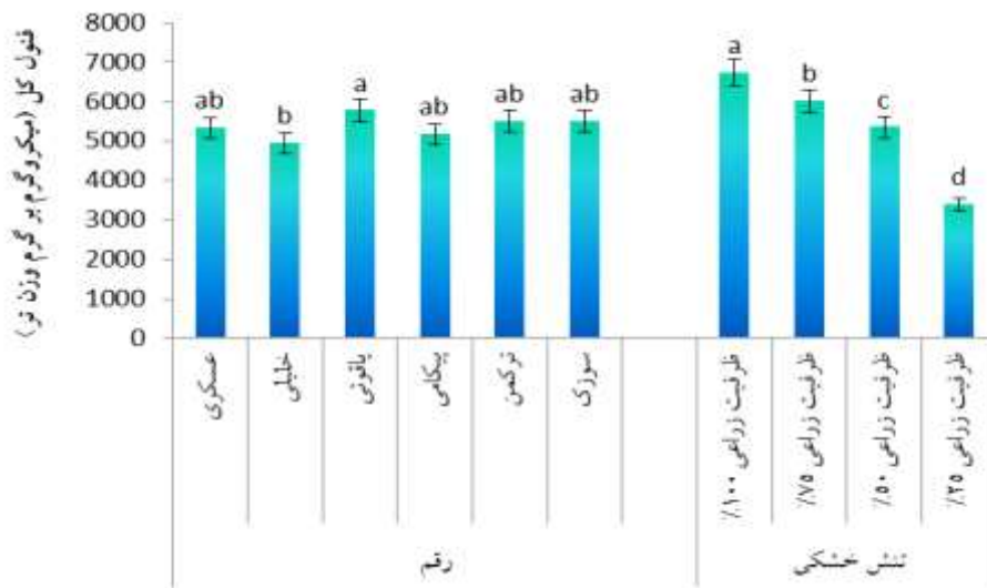
شکل ۱- میزان فنول کل در ارقام مختلف انگور تحت شرایط آبی متفاوت
