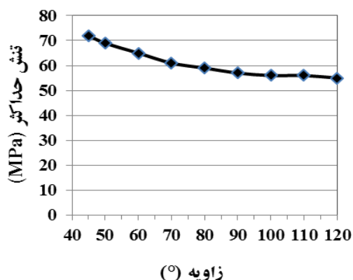
شکل (۸) روند تغییرات حداکثر تنش پد به ازای زوایای مختلف پروفیل در ضخامت پد و بارگذاری ثابت
