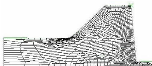
شکل (۱۰) وضعیت نهایی فضای داخلی قالب مدل شبیه‌سازی شده با مقادیر الگوریتم ژنتیک.
