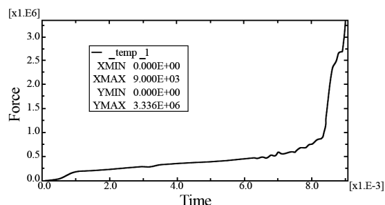
شکل (۹) نیروی فورج به دست آمده از مدل شبیه‌سازی شده با مقادیر کار تجربی.
