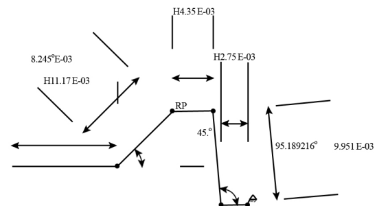
شکل (۳) شکل هندسی قالب.
