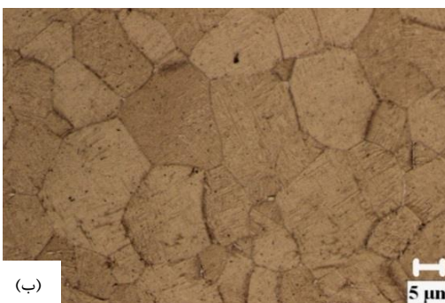
شکل (۳) ریزساختار نمونه آنیل انحلالی - کوئنچ و پیرسازی شده (الف): نمونه B و (ب): نمونه E.
