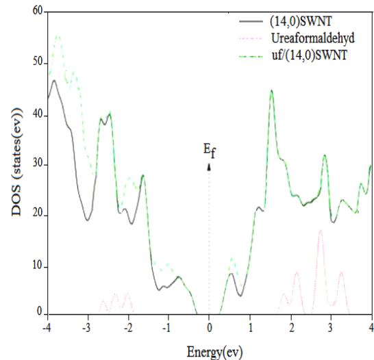
شکل (۵) DOS مربوط به نانولوله کربنی اولیه، سیستم نانولوله-کربنی (۱۴،۰) به همراه پلیمر اوره فرمالدهید و مونومر اوره فرمالدهید جذب شده.
