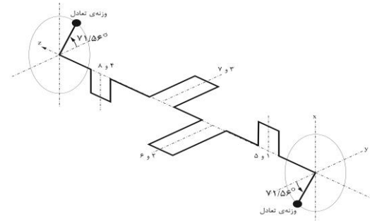
شکل (۱) استفاده از وزنه‌های تعادل چرخشی برای متعادل کردن نیروهای لرزشی در موتور هشت سیلندر خورجینی
