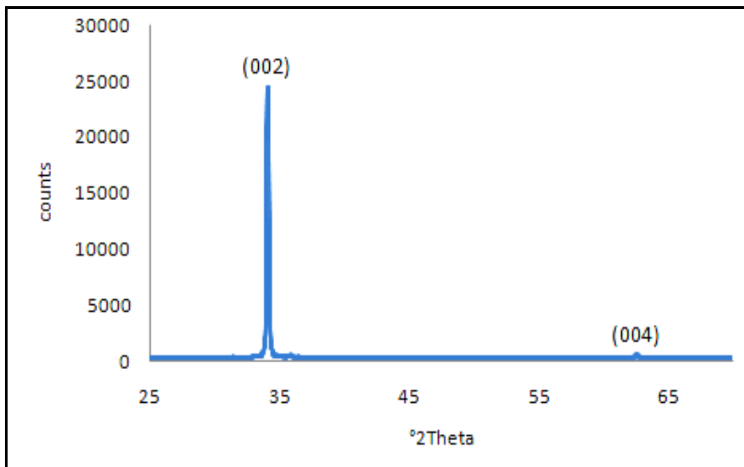
شکل (۴): نمودار حاصل از آنالیز XRD از پوشش نانو سیم همراستای اکسید روی.
