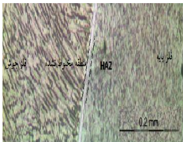
شکل (۱۱): تصویر میکروسکوپ نوری، فصل مشترک فلز پایه AISI 514 و فلز جوش 309L
