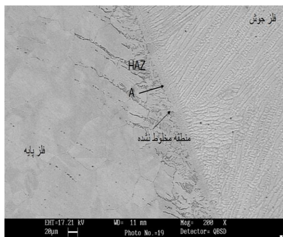
شکل (۱۵): تصویر میکروسکوپ الکترونی روبشی، فصل مشترک فلز 304L و فلز جوش ERNiCr-3
