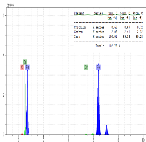
شکل (۱۳): نتایج آنالیز عنصری منطقه مخلوط نشده در مرز ذوب فلز پایه فولاد کونچ تمپر شده AISI 514 و فلز جوش 309L
