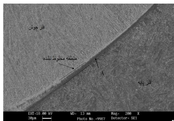
شکل (۱۲): تصویر الکترونی روبشی، ناحیه باریک در فصل مشترک فولاد کونچ تمپر شده AISI 514 و فلز جوش 309L
