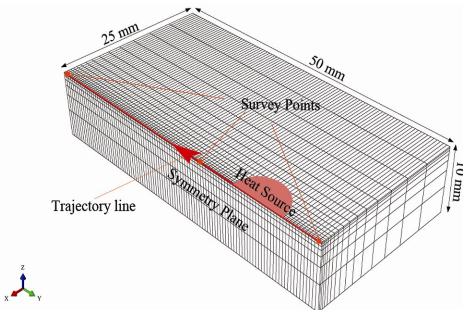
شکل (۱): نمای شماتیک فرآیند سخت گردانی استحاله ای بوسیله یک مسیر از حرکت منبع حرارتی متحرک
