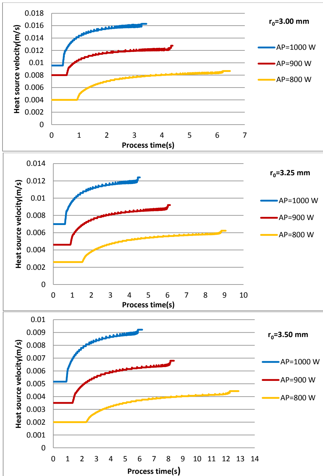
شکل (۳): پیش بینی تغییرات مورد نیاز در سرعت حرکت منبع حرارتی توسط تحلیل های اجزای محدود در حضور استراتژی کنترل سرعت برای شعاع های مختلف
