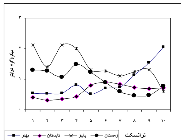
شکل ۶: تغییرات فصلی کدورت ترانسکت های مورد بررسی
