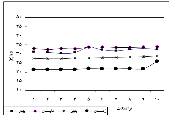
شکل ۱: تغییرات فصلی دما در ترانسکت های مورد بررسی
