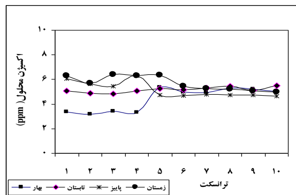
شکل ۴: تغییرات فصلی اکسیژن اشباع ترانسکت های مورد بررسی
