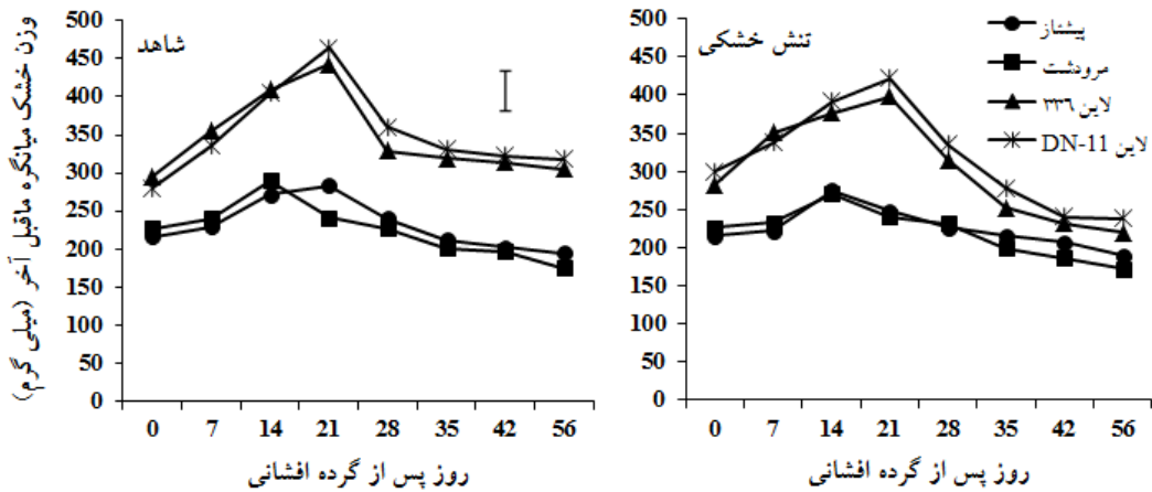
شکل ۳- روند تغییرات وزن خشک و غلظت قندهای محلول میانگه دم گل آذین چهار ژنوتیپ گندم مورد بررسی پس از گرده افشانی در شرایط شاهد و تنش خشکی. I: شاخص LSD ( \alpha=0.05 ) نشان دهنده تفاوت‌های معنی‌دار می‌باشد
