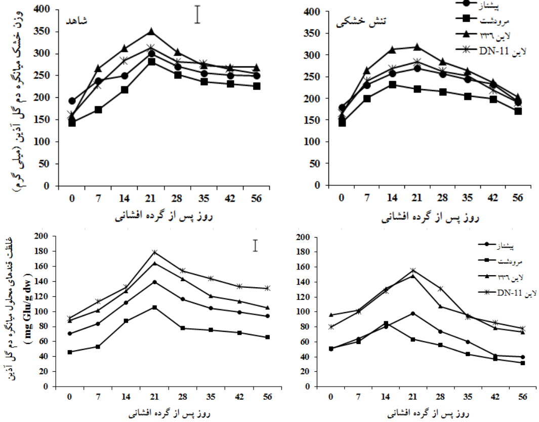
شکل ۳- روند تغییرات وزن خشک و غلظت قندهای محلول میانگه دم گل آذین چهار ژنوتیپ گندم مورد بررسی پس از گرده افشانی در شرایط شاهد و تنش خشکی. I: شاخص LSD ( \alpha=0.05 ) نشان دهنده تفاوت‌های معنی‌دار می‌باشد
