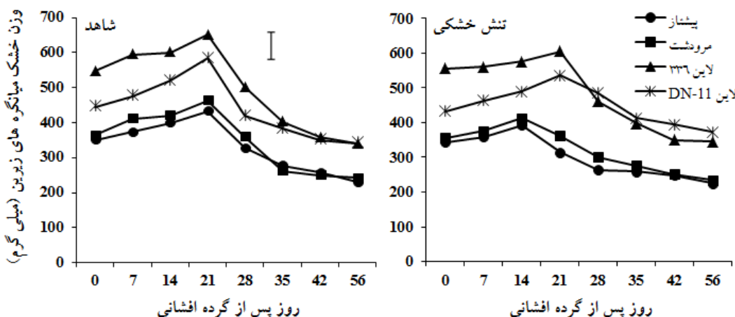
شکل ۴- روند تغییرات وزن خشک و غلظت قندهای محلول میانگه ماقبل آخر چهار ژنوتیپ گندم مورد بررسی پس از گرده افشانی در شرایط شاهد و تنش خشکی. I: شاخص LSD ( \alpha=0.05 ) نشان دهنده تفاوت‌های معنی‌دار می‌باشد
