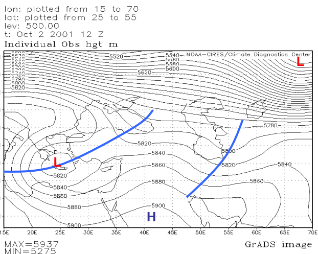
شکل ۲۱ : نقشه سطح ۵۰۰ هکتوپاسکال ساعت ۱۲ روز دوم اکتبر ۲۰۰۱
