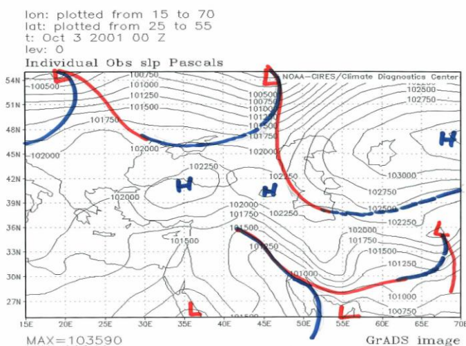
شکل ۲۳ : نقشه سطح زمین ساعت ۰۰ روز سوم اکتبر ۲۰۰۱ و موقعیت جبهه های سطح زمین
