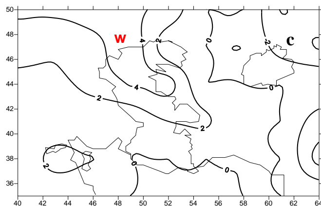
شکل ۲۲: میدان فرارفت دما در ساعت ۱۲ روز دوم اکتبر ۲۰۰۱ (بوسیله باد سطح ۱۰۰۰ هکتوپاسکال) - واحد خطوط هم‌مقدار
