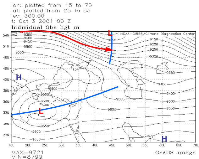
شکل ۲۷ : نقشه سطح ۳۰۰ هکتوپاسکال ساعت ۰۰ روز سوم اکتبر ۲۰۰۱
