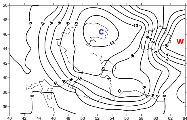
شکل ۲۸ : میدان فرارفت دما در ساعت ۱۲ روز اول اکتبر ۲۰۰۱ ( بوسیله باد سطح ۷۰۰ هکتوپاسکال ) - واحد
