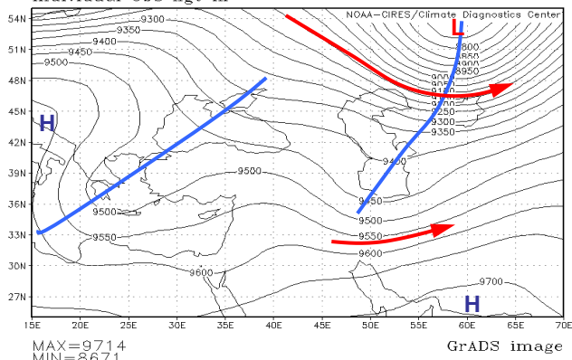
شکل ۱۷ : نقشه سطح ۳۰۰ هکتوپاسکال ساعت ۰۰ روز دوم اکتبر ۲۰۰۱
