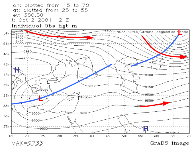
شکل ۲۲ : نقشه سطح ۳۰۰ هکتوپاسکال ساعت ۱۲ روز دوم اکتبر ۲۰۰۱
