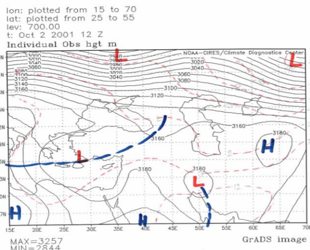
شکل ۲۰ : نقشه سطح ۷۰۰ هکتوپاسکال ساعت ۱۲ روز دوم اکتبر ۲۰۰۱ و توزیع میدان دما در سطح ۷۰۰
