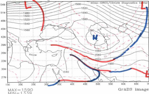
شکل ۱۴: نقشه سطح ۸۵۰ هکتوپاسکال ساعت ۰۰ روز دوم اکتبر ۲۰۰۱ و توزیع میدان دما و موقعیت جبهه ها در سطح ۸۵۰ هکتوپاسکال
