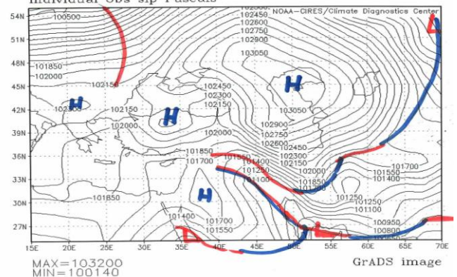
شکل ۱۳: نقشه سطح زمین ساعت ۰۰ روز دوم اکتبر ۲۰۰۱ و موقعیت جبهه های سطح زمین
