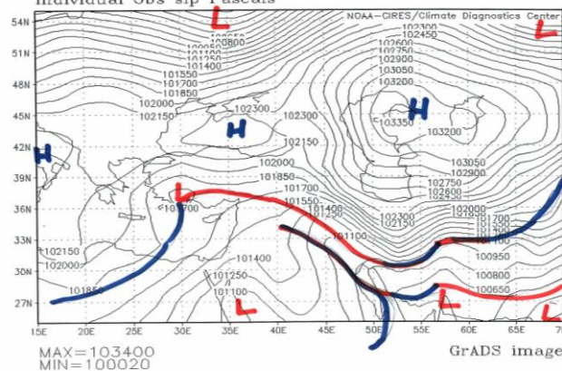
شکل ۱۸ : نقشه سطح زمین ساعت ۱۲ روز دوم اکتبر ۲۰۰۱ و موقعیت جبهه های سطح زمین
