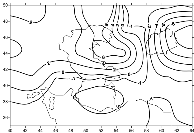
شکل ۲۹ : میدان فرارفت دما در ساعت ۰۰ روز دوم اکتبر ۲۰۰۱ ( بوسیله باد سطح ۷۰۰ هکتوپاسکال ) - واحد خطوط هم‌مقدار ^{\circ}\text{C}/12\text{h}
