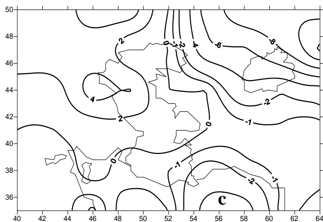
شکل ۳۱ : میدان فرارفت دما در ساعت ۱۲ روز دوم اکتبر ۲۰۰۱ ( بوسیله باد سطح ۷۰۰ هکتوپاسکال ) - واحد خطوط هم‌مقدار ^{\circ}\text{C}/12\text{h}
