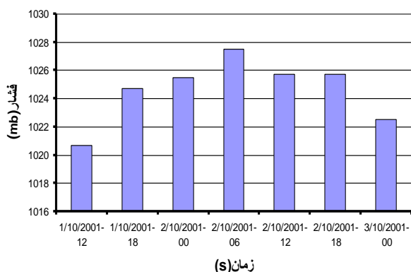
شکل ۷- نمودار تغییرات فشار در مدت ۳۶ ساعت در نوشهر در اکتبر ۲۰۰۱
