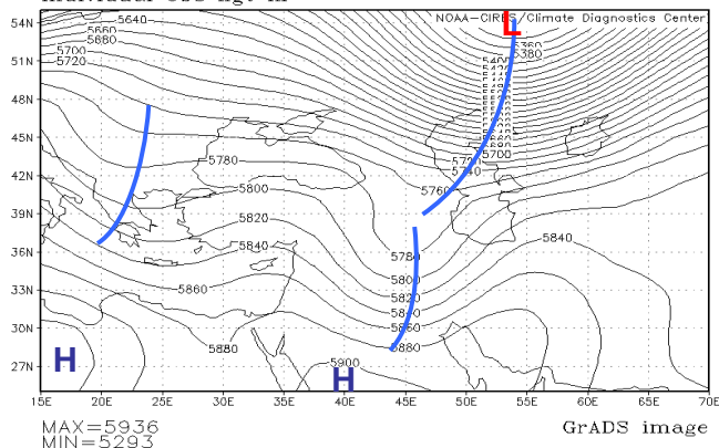
شکل ۱۱: نقشه سطح ۵۰۰ هکتوپاسکال ساعت ۱۲ روز اول اکتبر ۲۰۰۱
