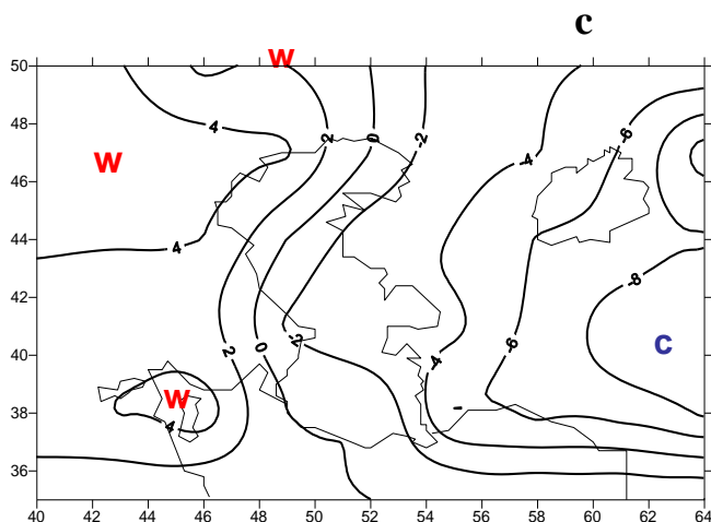
شکل ۳۰ : میدان فرارفت دما در ساعت ۰۰ روز دوم اکتبر ۲۰۰۱ ( بوسیله باد سطح ۱۰۰۰ هکتوپاسکال ) - واحد خطوط هم‌مقدار
