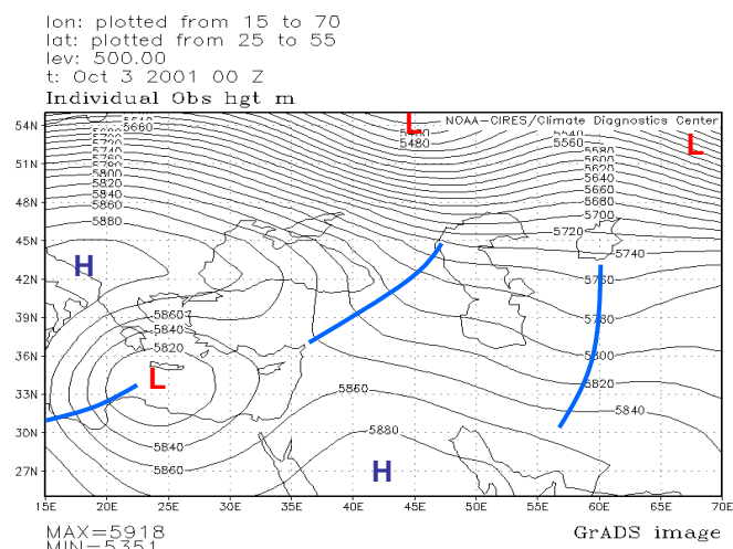
شکل ۲۶ : نقشه سطح ۵۰۰ هکتوپاسکال ساعت ۰۰ روز سوم اکتبر ۲۰۰۱
