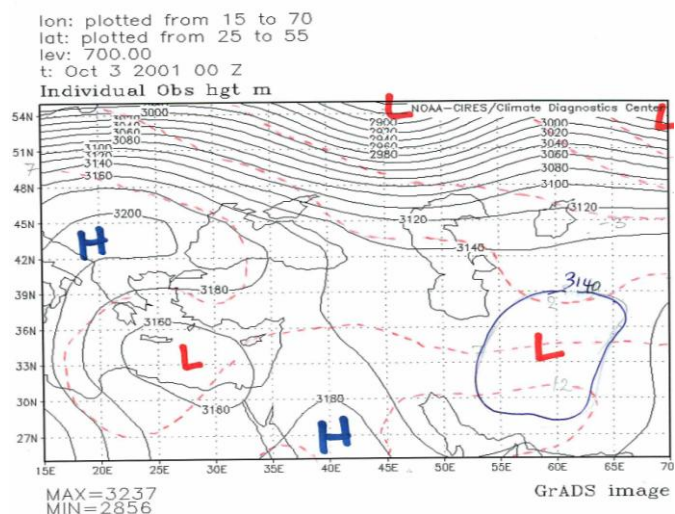
شکل ۲۵ : نقشه سطح ۷۰۰ هکتوپاسکال ساعت ۰۰ روز سوم اکتبر ۲۰۰۱ و توزیع میدان دما در سطح ۷۰۰ هکتوپاسکال
