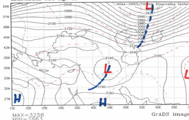
شکل ۱۰: نقشه سطح ۷۰۰ هکتوپاسکال ساعت ۱۲ روز اول اکتبر ۲۰۰۱ و توزیع میدان دما در سطح ۷۰۰ هکتوپاسکال
