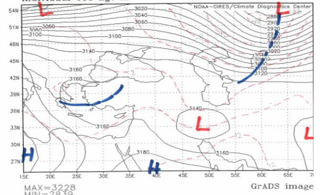
شکل ۱۵: نقشه سطح ۷۰۰ هکتوپاسکال ساعت ۰۰ روز دوم اکتبر ۲۰۰۱ و توزیع میدان دما در سطح ۷۰۰
