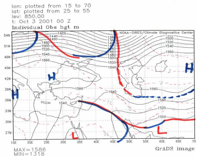
شکل ۲۴ : نقشه سطح ۸۵۰ هکتوپاسکال ساعت ۰۰ روز سوم اکتبر ۲۰۰۱ و توزیع میدان دما و موقعیت جبهه ها در سطح ۸۵۰ هکتوپاسکال
