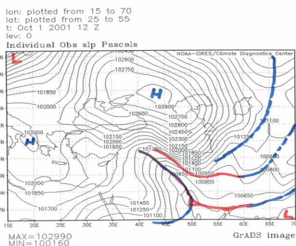
شکل ۸ : نقشه سطح زمین ساعت 12 روز اول اکتبر 2001 و موقعیت جبهه های سطح زمین
