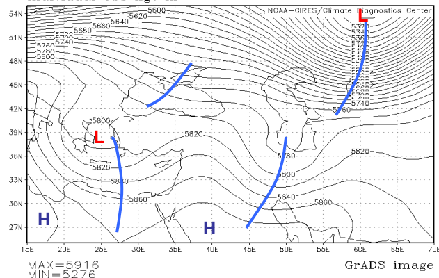
شکل ۱۶ : نقشه سطح ۵۰۰ هکتوپاسکال ساعت ۰۰ روز دوم اکتبر ۲۰۰۱
