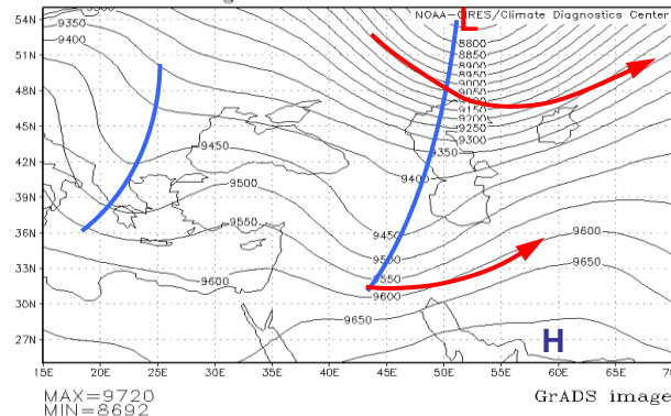
شکل ۱۲: نقشه سطح ۳۰۰ هکتوپاسکال ساعت ۱۲ روز اول اکتبر ۲۰۰۱
