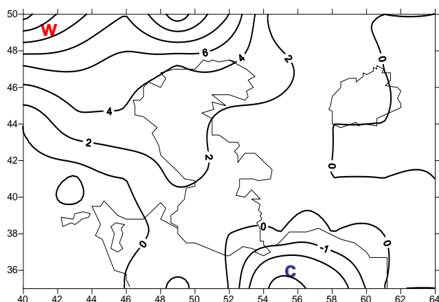
شکل ۲۳: میدان فرارفت دما در ساعت ۰۰ روز سوم اکتبر ۲۰۰۱ (بوسیله باد سطح ۷۰۰ هکتوپاسکال) -
