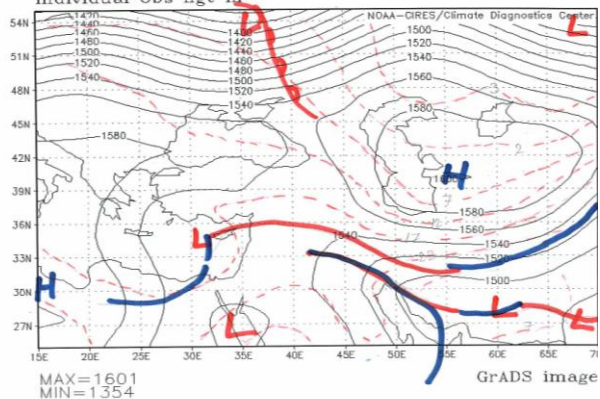
شکل ۱۹ : نقشه سطح ۸۵۰ هکتوپاسکال ساعت ۱۲ روز دوم اکتبر ۲۰۰۱ توزیع میدان دما و موقعیت جبهه ها در
