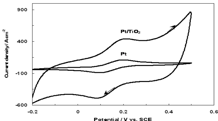
شکل ۳ منحنی ولتامتری چرخه ای الکترو پلاتین در محلولی حاوی ۱ مول پتاسیم کلرید و ۱۰ میلی مول پتاسیم فری سیانید با سرعت روبش ۵۰ mV/s
