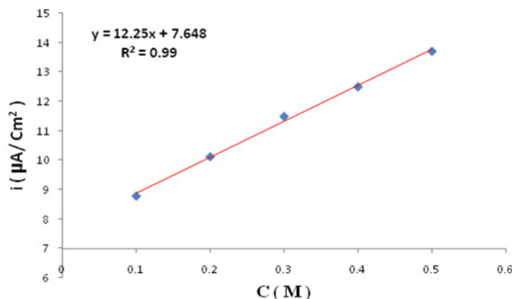
شکل ۸ نمودار جریان بیک اکسایش گلوکز بر روی الکترود Pt/TiO 2 /Ti برحسب غلظت گلوکز
