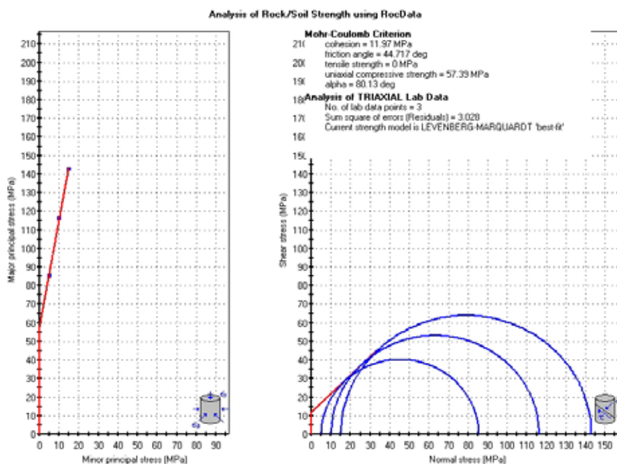
تصویر ۸- دایره موهر رسم شده در سه سطح تنش مورد آزمایش توسط نرم افزار RocData
