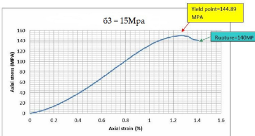
تصویر ۵- نمودار تنش- کرنش آزمون سه محوری در تنش جانبی ۱۵ (Mpa)
