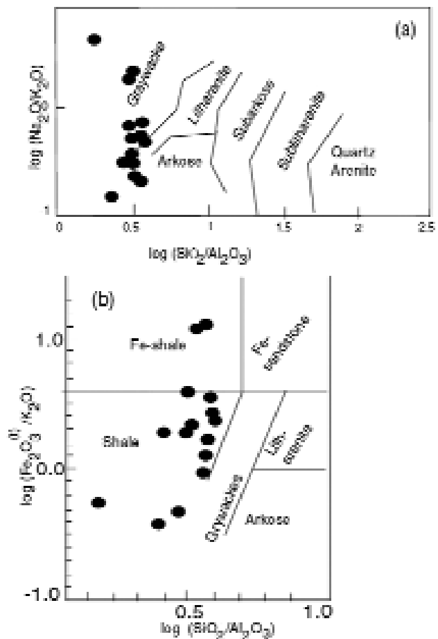
تصویر ۵- طبقه‌بندی پتی جان و همکاران (Pettijohn et al. 1972)، مرزها توسط هرون (Herron 1988) اصلاح شده است. طبق این نمودار اکثر متاپلیت‌های ماهنشان از نوع گریوک می‌باشند. b- طبقه‌بندی هرون (Herron 1988) که بر اساس آن متاپلیت‌ها از نوع شیل می‌باشند.
