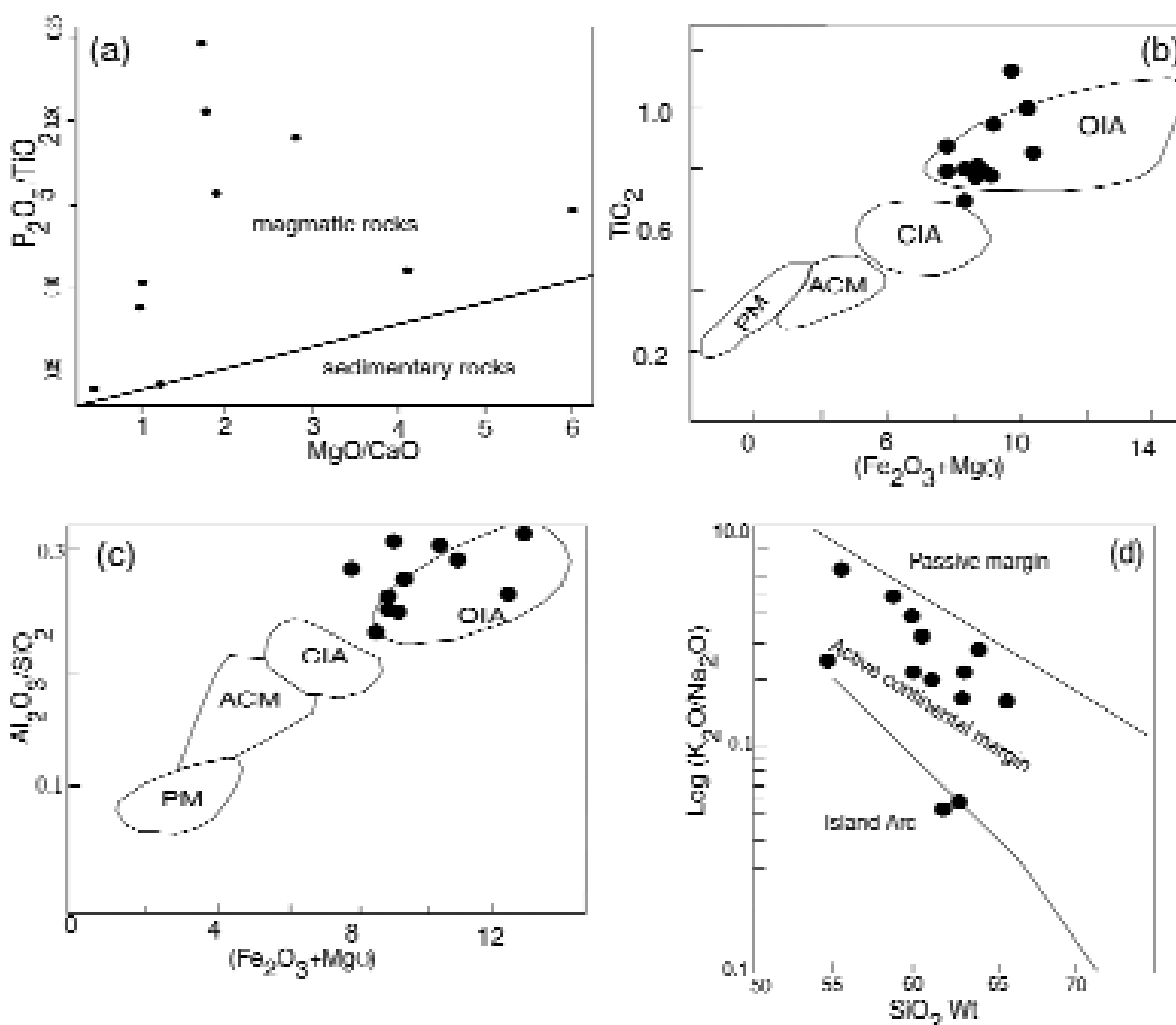
تصویر a-v- نمودار دوتایی MgO/CaO در مقابل P 2 O 5 /TiO 2 در این نمودار سنگ‌های ماگمایی اسیدی از سنگ‌های رسوبی دگرگون شده متمایز شده‌اند، به عبارتی ارتو و یا پارا بودن منشاء آن‌ها مشخص شد، b و c- نمودارهای باتیا (Bhatia 1983) که طبق آن نمونه‌های متاپلیتی ماهنشان در محدوده‌ی جزایر قوس اقیانوسی (Oceanic Island Arc: OIA) قرار گرفته‌اند. d- بر اساس نمودار روزر و کورش (1986) Roser & Korsch (1998) نمونه‌ها در محدوده‌ی حاشیه‌ی فعال قاره‌ای و مرتبط با قوس آتشفشانی قرار گرفته‌اند. PM: Passive Margin, CIA: Continental Volcanic Arc, ACM: Active Continental Margin,
