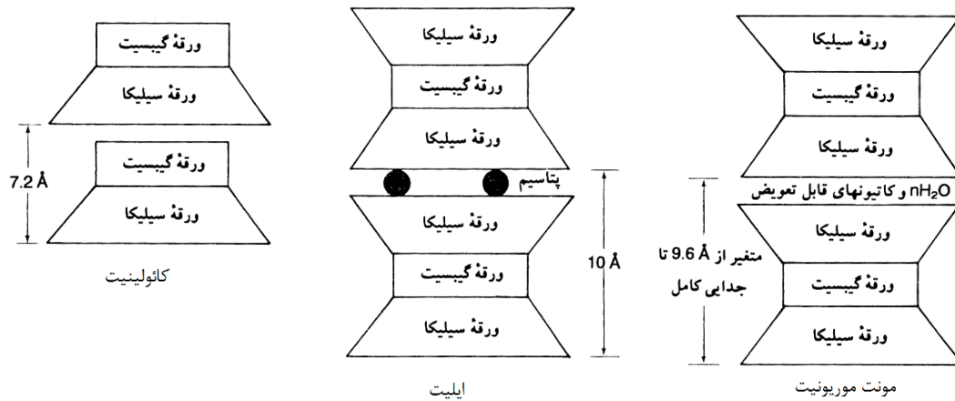
تصویر ۲- نمودار ساختمانی (الف) کائولینیت، (ب) ایلیت و (پ) مونت مورینونیت (طاهونی ۱۳۷۶).
