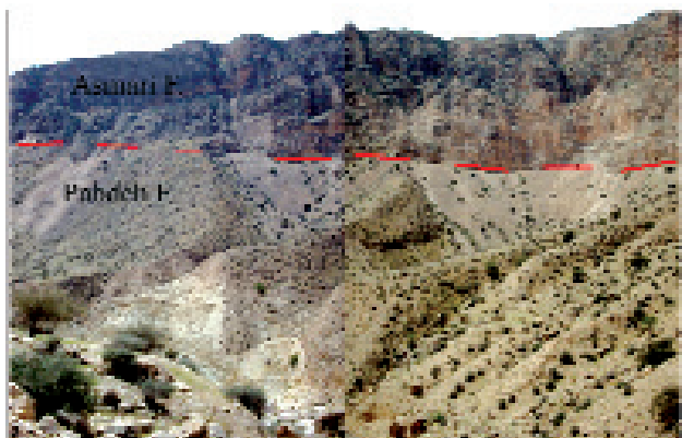
تصویر ۳- دور نمایی از سازندهای پایده و آسماری (نگاه به سمت جنوب غرب)
