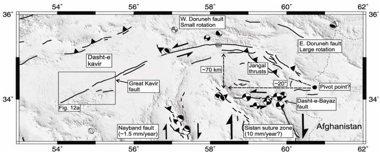
تصویر ۱۸- نقشی که گسل بزرگ کویر یا درونه در تکتونیک شرق ایران ایفا می‌کند. ژئومورفولوژی شرق میکروپلیت ایران متأثر از عملکرد این گسل بزرگ می‌باشد (Farhoudi 1991). گسل چپ‌گرد درونه با طولی در حدود ۶۵۰ کیلومتر یکی از بزرگ‌ترین گسل‌های شرق ایران است (Walker & Jackson 2004).
