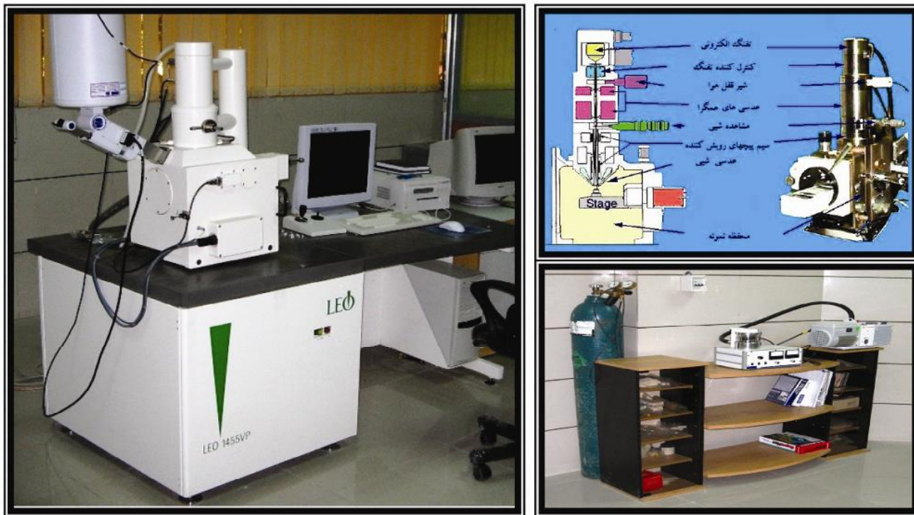
تصویر ۳- نمایی از دستگاه میکروسکوپ الکترونی روبشی مدل Leo 1455 VP (با قابلیت آنالیز توسط طیف اشعه ایکس) همراه با ساختار داخلی، اصول و سیستم آماده سازی نمونه (Ag-Coating) مورد استفاده در این پژوهش را نشان می‌دهند.
