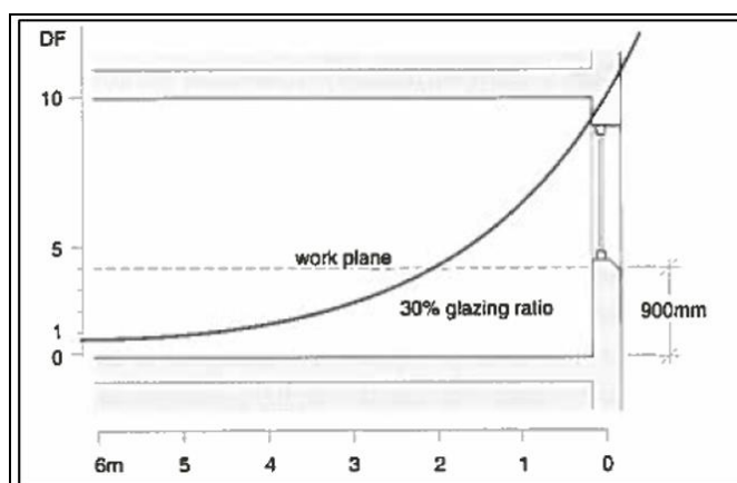
شکل ۴- افت سریع DF با فاصله از دیوار پنجره
