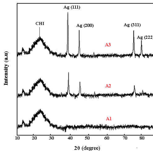
شکل ۱- الگوی پراش اشعه X کیتوسان (A 1 ) و نانو بایو کامپوزیت نقره/کیتوسان در غلظت‌های مختلف نیترات نقره، (A 2 ): ۰/۱۵ mol/L و (A 3 ): ۰/۱۵ mol/L
