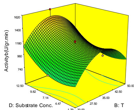
شکل ۸- اثر دما و غلظت سوبسترا بر فعالیت آنزیمی
