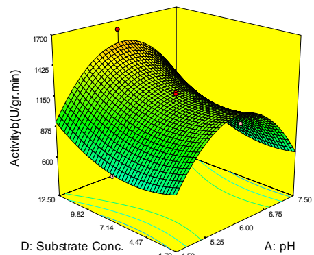
شکل ۶- اثر غلظت سوبسترا و pH بر فعالیت آنزیمی
