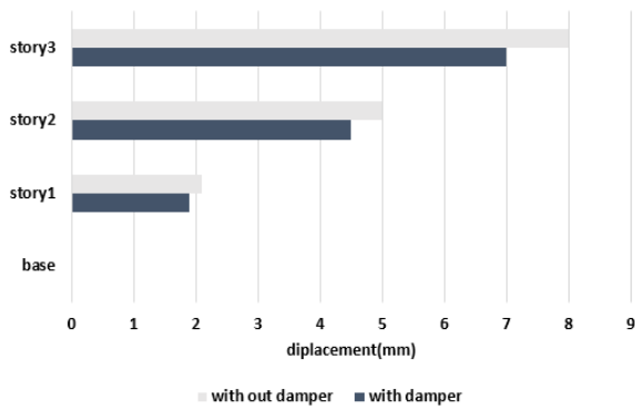
الف) جابجایی طبقات در قاب سه طبقه
