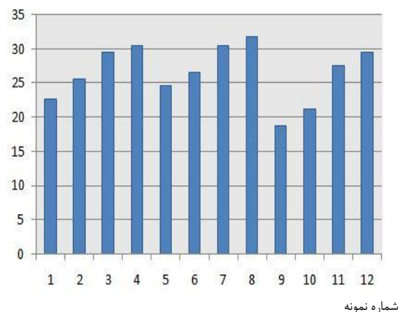
شکل ۱- نمودار درصد تخلخل
