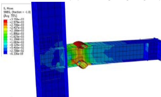
شکل ۷- منحنی میزان تنش در مدل DAFS1
