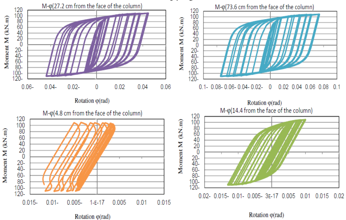
شکل ۹- منحنی لنگر خمشی تیر در وجه اتصال به ستون به زاویه تغییر مکان نسبی در نقاط مختلف تیر در مدل AFS2 با ضخامت 1.2 cm جهت مقاطع کمانی معکوس استفاده شده
